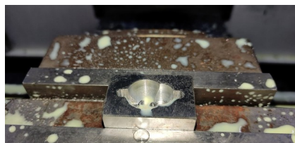
Formverktyg uppspönt i maskin
