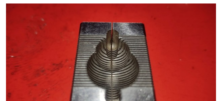
Formverktyg, kylflänspaket
